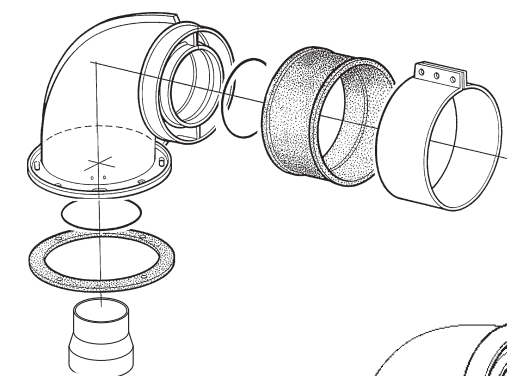
Coude de sortie coaxial (1KWMA31K)
